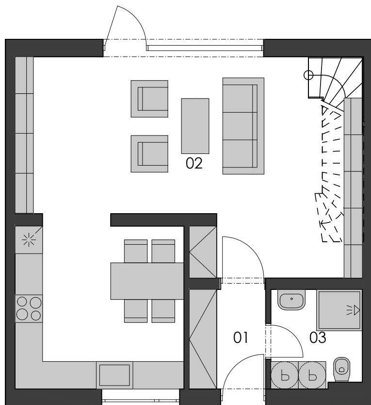
Půdorys domu
