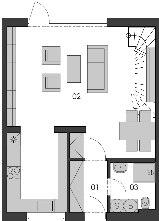
Půdorys domu
